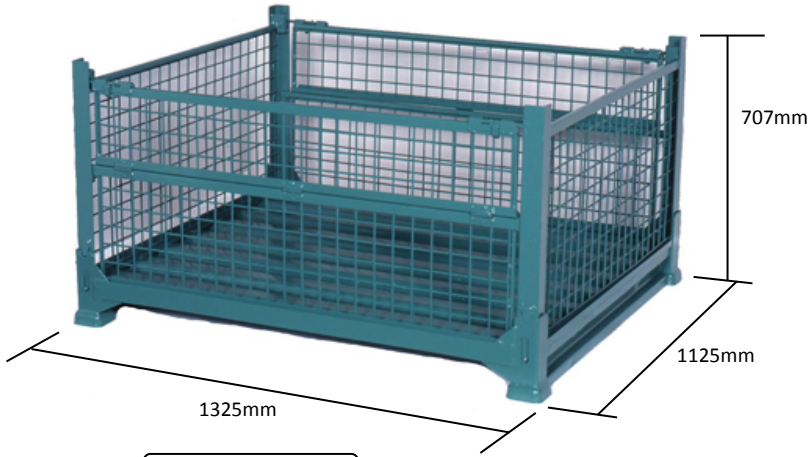
組立状態
